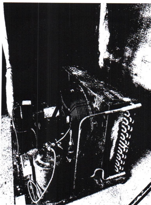
03- Parte da lateral direita da unidade condensadora da câmara frigorífica (resfriamento).
