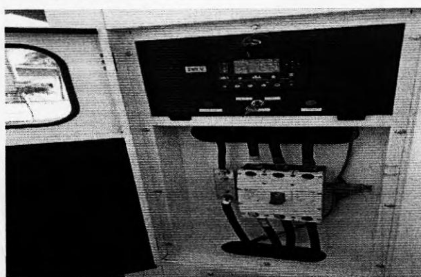
Quadro e chave controladora
