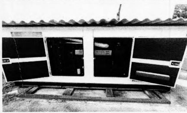
Compartimento do motor (retaguarda)
