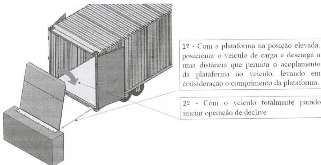
Figura 14: posicionamento do veículo de carga
