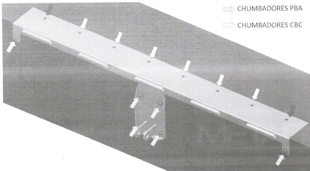
Figura 4: Pontos de aplicação dos chumbadores.
