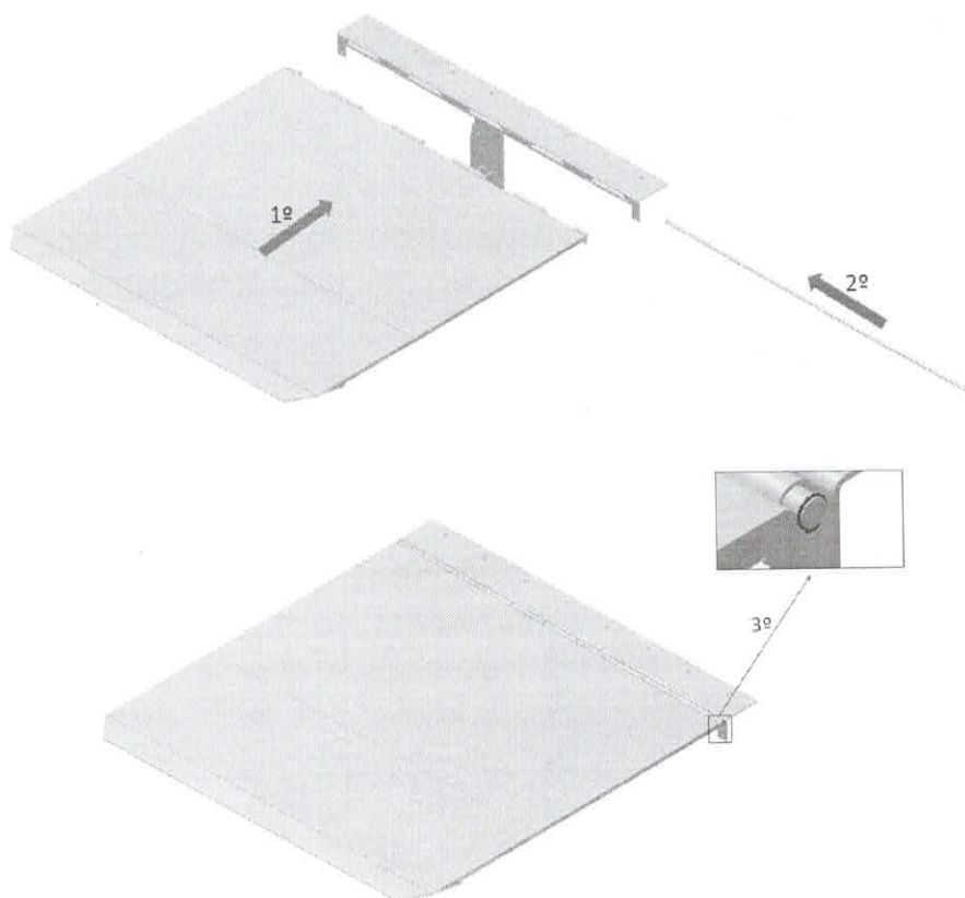
Figura 6: Montagem do eixo principal
