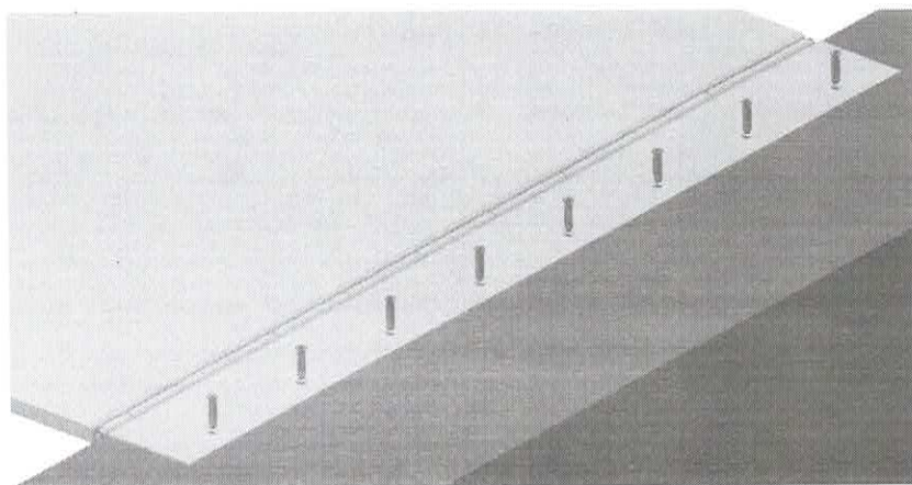
Figura 8: Posicionamento dos chumbadores nos furos e aperto
