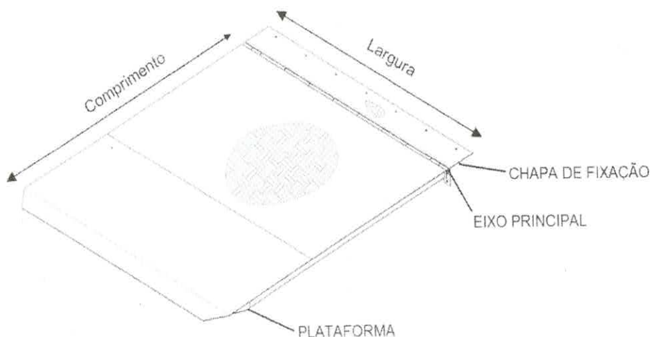
Figura 1: Dimensões da plataforma niveladora de doca avançada.
