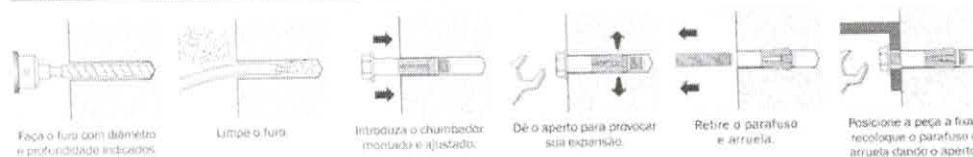
Figura 5: Orientações para aplicação dos chumbadores CBC (Fonte: Âncora, 2017).
