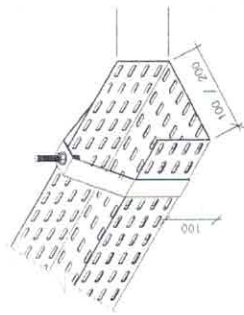
DET. 4 - ELETROCALHA COM SUSPENSÃO VERTICAL
