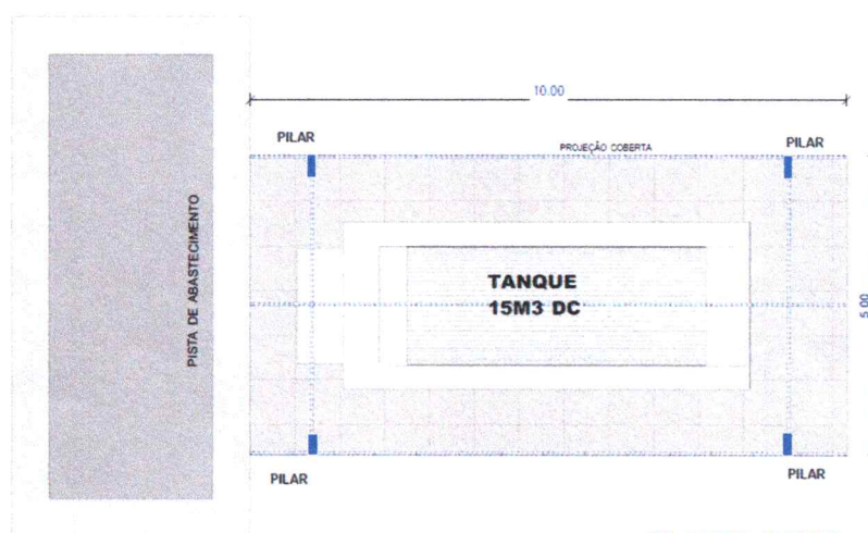
PLANTA BAIXA ESCALA 1:50
