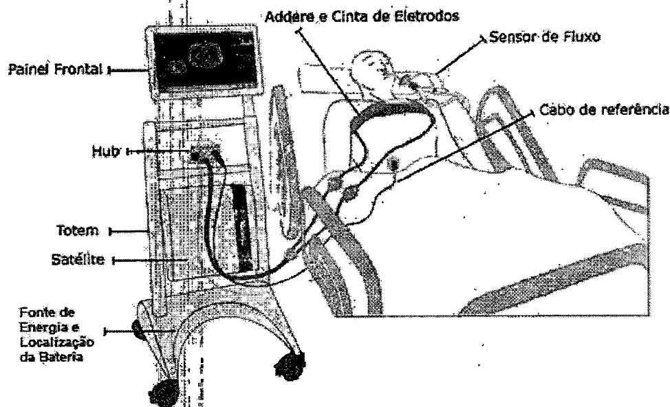
Figura 8 – Visão Geral
