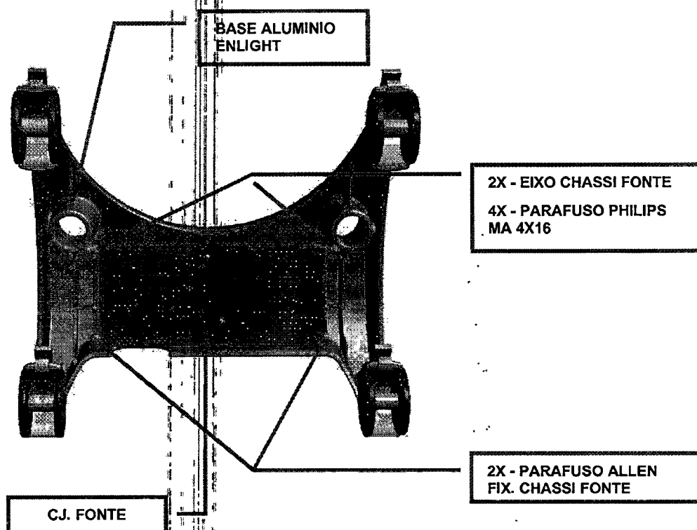
Figura 33 - Vista inferior do Enlight 1800 MAX
